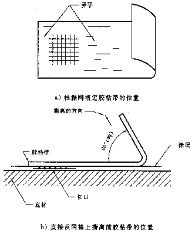
图3 胶粘带的定位
