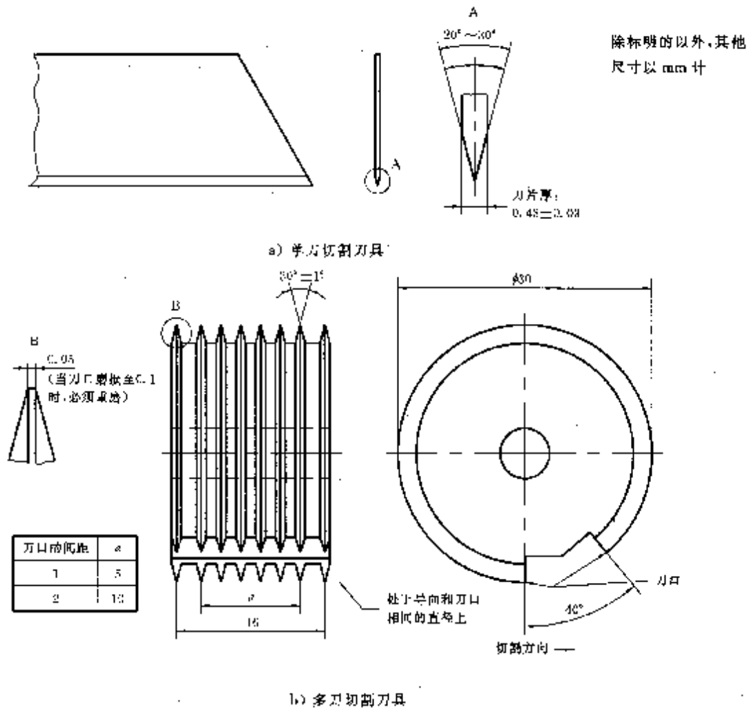
图 1 适合的切割刀具
